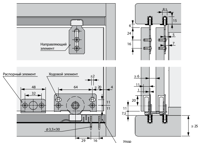
Монтажная схема, поперечное сечение
