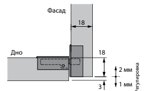
Петля для откидных фасадов Markant 11
