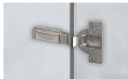
Специальная петля для толщины фасада до 43 мм.
