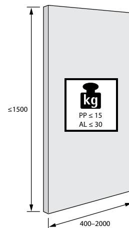
Размеры и вес двери
