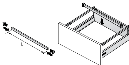
Монтажная схема
