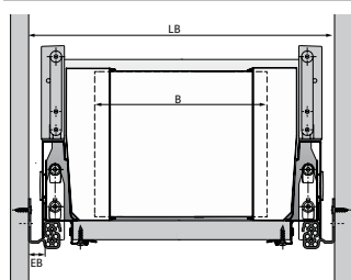
Схема раскроя поперечного разделителя OrgaStore 820 (Atira)
