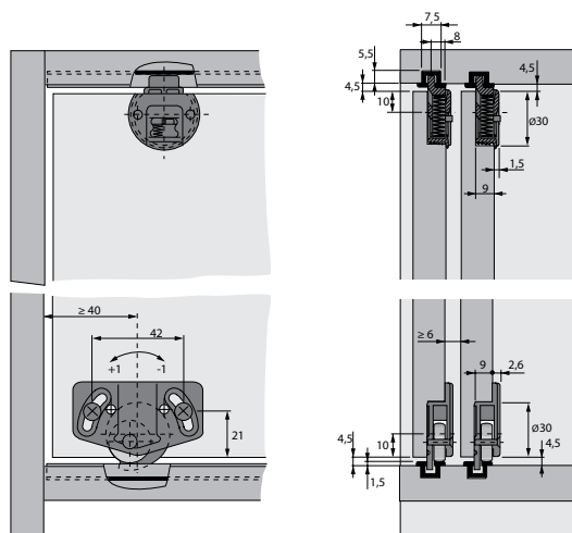
Монтажная схема, поперечное сечение
