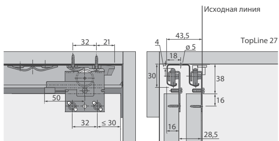
Монтажная схема, поперечное сечение
