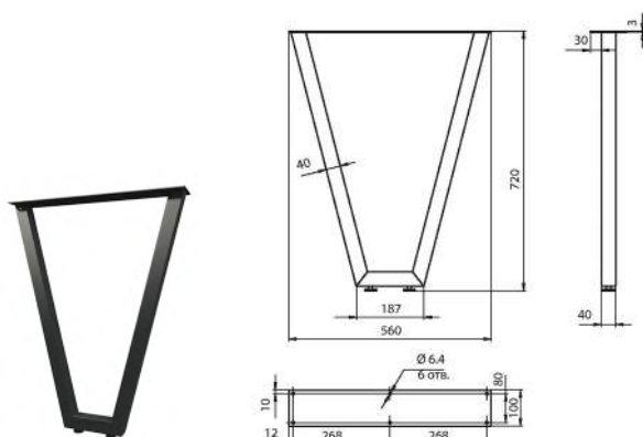
Опора для стола ЛИССАБОН
