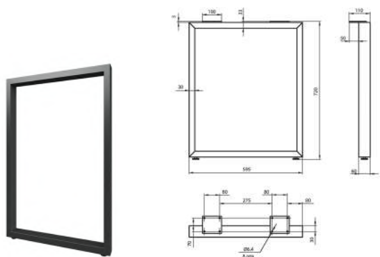
Опора для столешницы МАДРИД
