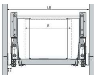
Схема раскроя поперечного разделителя OrgaStore 820 (Atira)
