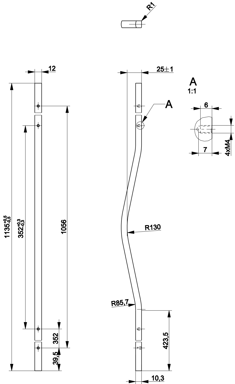
Uchwyt na profilu C-3690 Rozwinięcie L=1140 mm bez naddatku (potwierdzić w przyrządzie docelowym).
