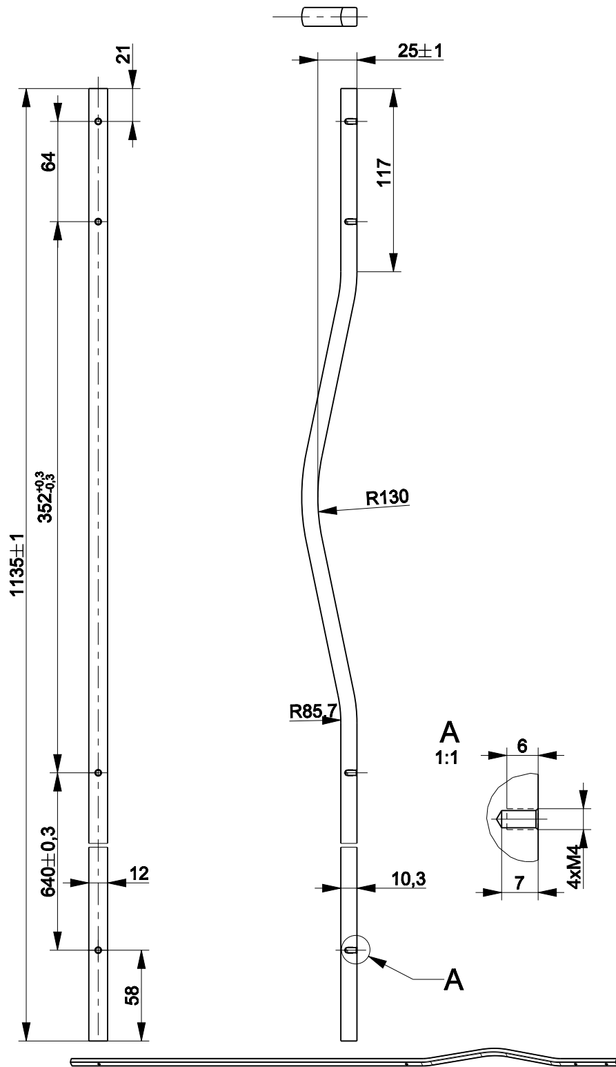
Uchwyt na profilu C-3690 Rozwinięcie L=1140 mm bez nadatku (potwierdzić w przyrządzie docelowym).
